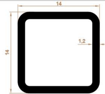
14x14 Emniyet Şeridi 14x14 Safety Strip
