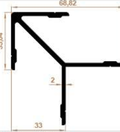
Aldoks (Orta) Köşe Takozu Aldox (Medium) Corner Wedge
