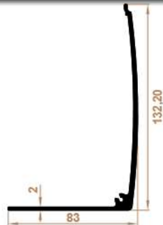
Üst Kasa Kapak Profili Upper Case Cover Profile
