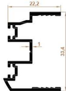
Açılı Dönüş Mentеше Profil PopUp Return Hinge Profile
