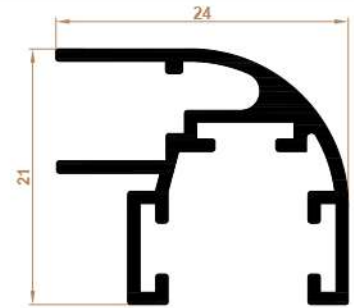
Köşe Dönüş Fitil Corner Return Wick
