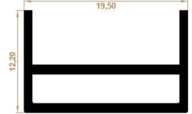
Slim Eşiksiz Profil Slim Profile without Threshold
