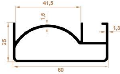
60x25 mm Üst Küpeşte Yandan Kanallı 60x25 mm Upper Handrail with Side Channel
