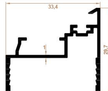
Sabit Cam Kilit Karşılığı Profil Stable Glass Lock Prevention Profile
